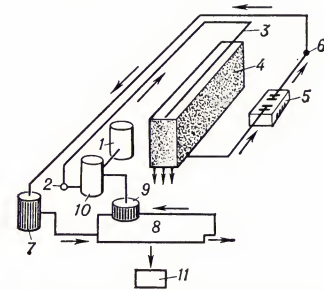
Рис. 2. Схема подземного выщелачивания скальных руд: 1 — емкость для растворятеля; 2 — насос; 3 — трубопровод рабочих растворов; 4 — отработываемый блок руды; 5 — емкость для сбора продуктивных растворов; 6 — насос; 7 — емкость для продуктивных растворов на поверхности; 8 — сорбционная установка; 9 — отстойник отработанного раствора; 10 — емкость для доукрепления растворов; 11 — пресс-фильтр.
